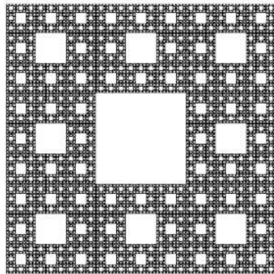
TAPETE DE SIERPINSKI
