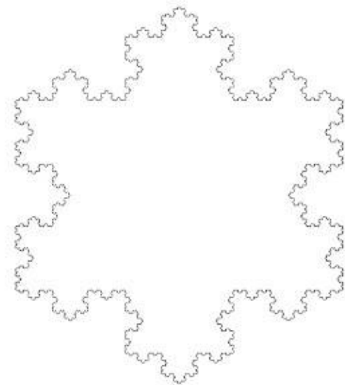
Copo de Koch
