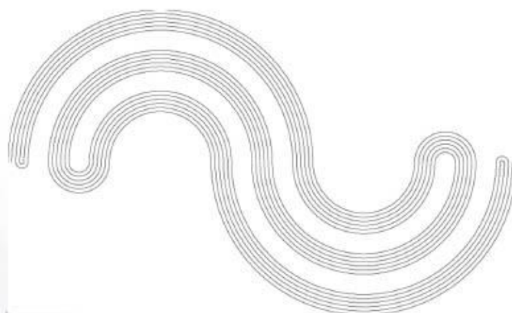
Continuo de Knaster
